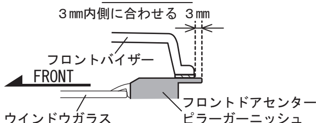
断面 d-d'
