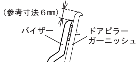
断面 g-g'
