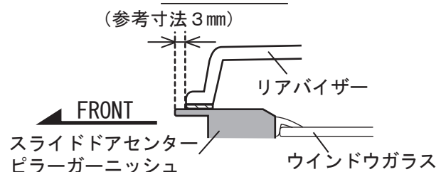
断面 g-g'
